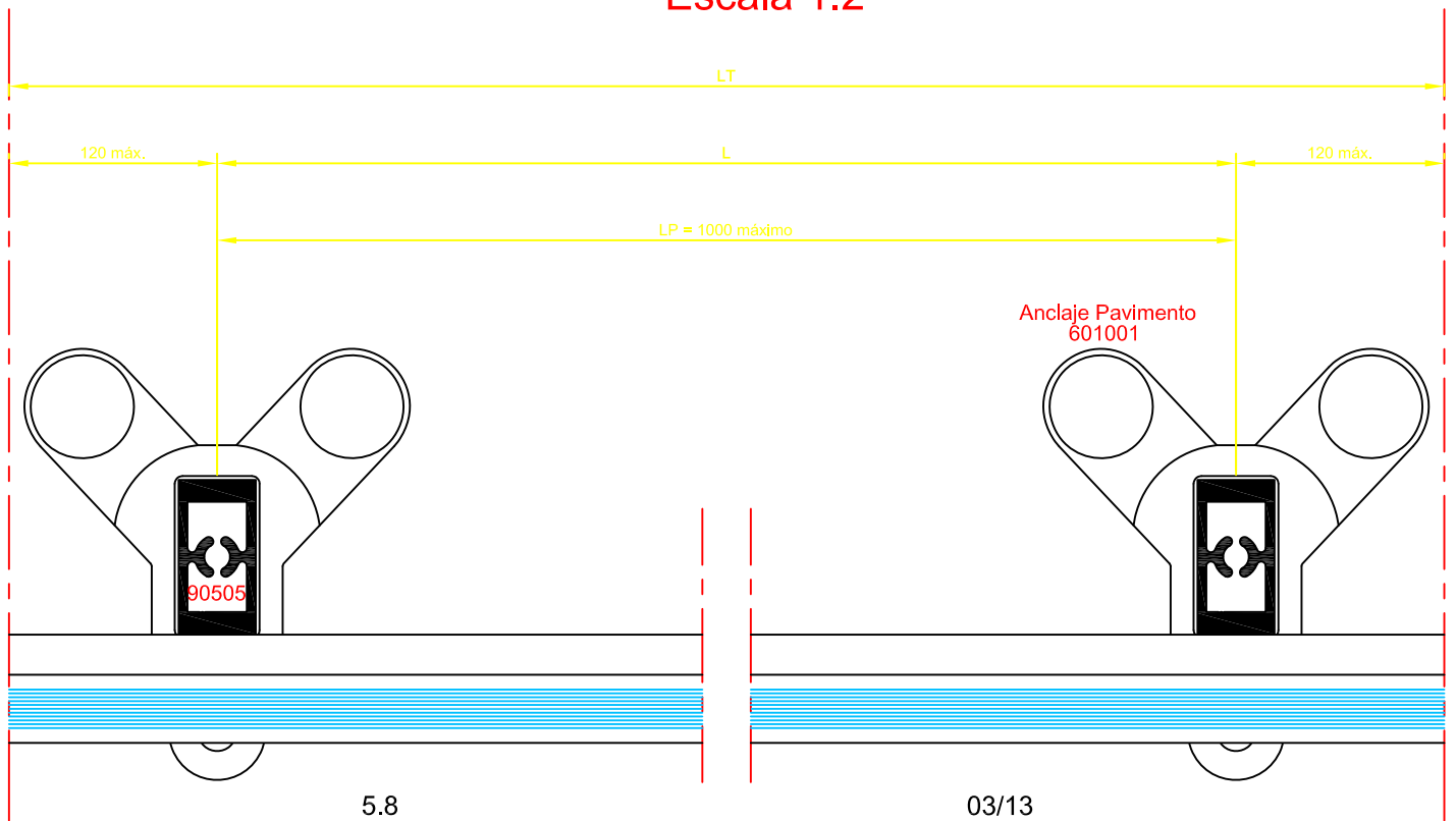
Sección Horizontal A-A' Escala 1:2
