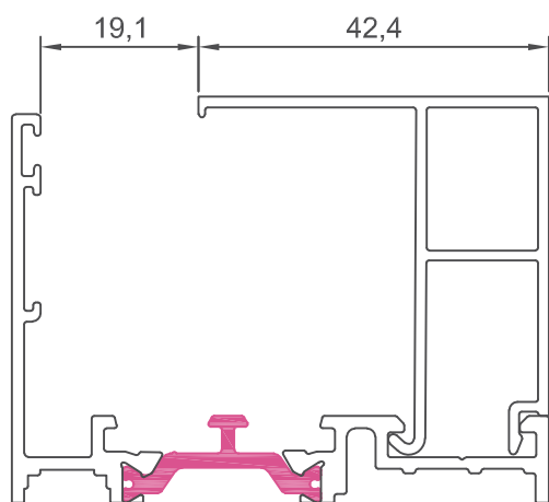
60543 junquillo 42,4 mm
