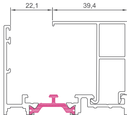
60542 junquillo 39,4 mm
