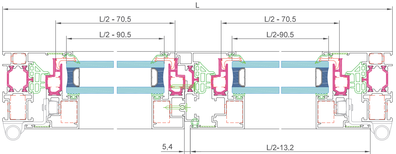
Escala Sección 1:2
