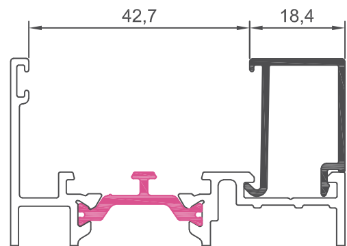
10004 junquillo 18,4 mm
