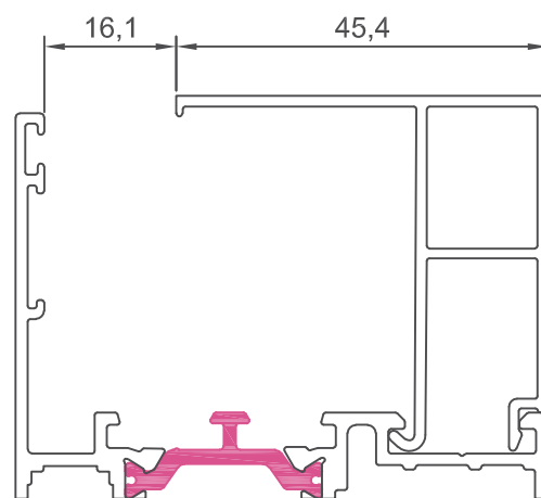
60544 junquillo 45,4 mm
