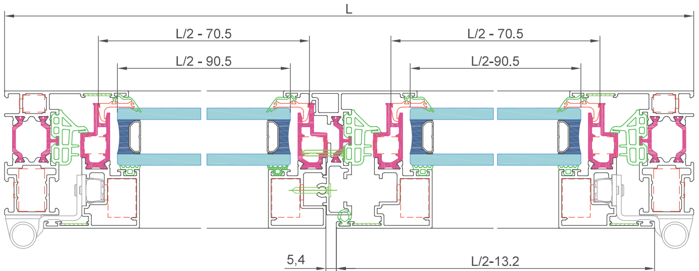
Escala Sección 1:2
