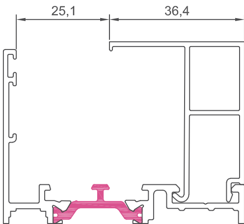
60541 junquillo 36,4 mm
