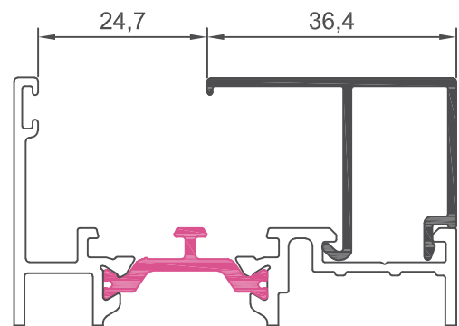
10010 junquillo 36,4 mm
