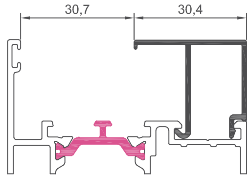
10008 junquillo 30,4 mm
