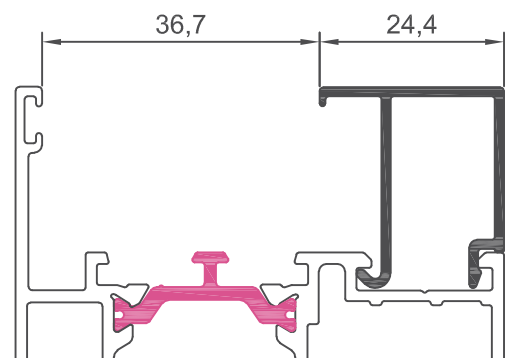
10006 junquillo 24,4 mm
