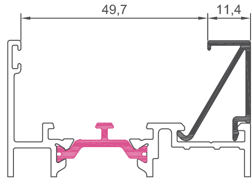
10002 junquillo 11,4 mm
