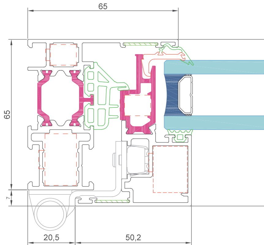
sección 3
