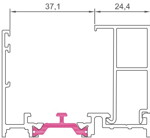
60536 junquillo 24,4 mm
