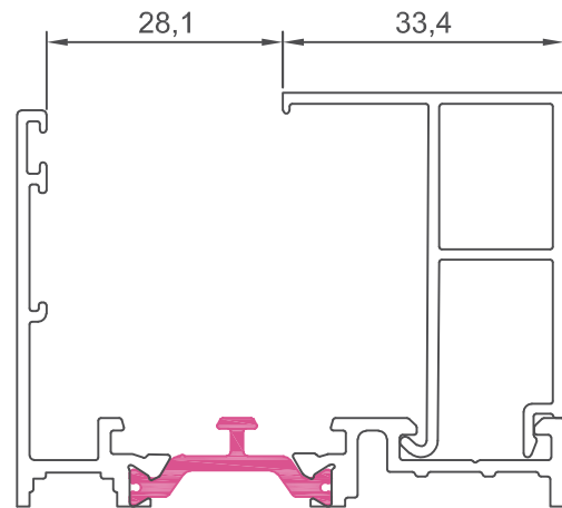
60539 junquillo 33,4 mm
