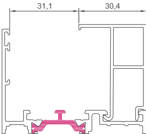
60538 junquillo 30,4 mm
