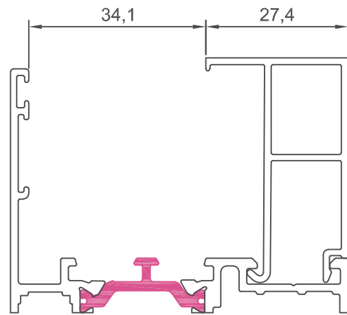
60537 junquillo 27,4 mm
