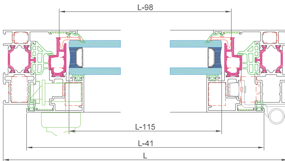
Escala Sección 1:2
