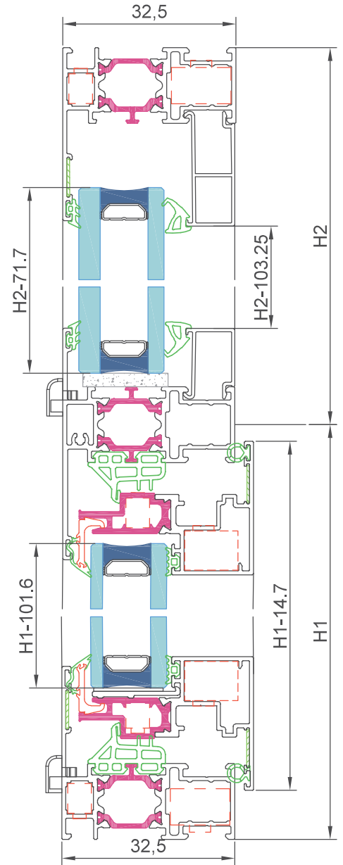
Escala 1:2
