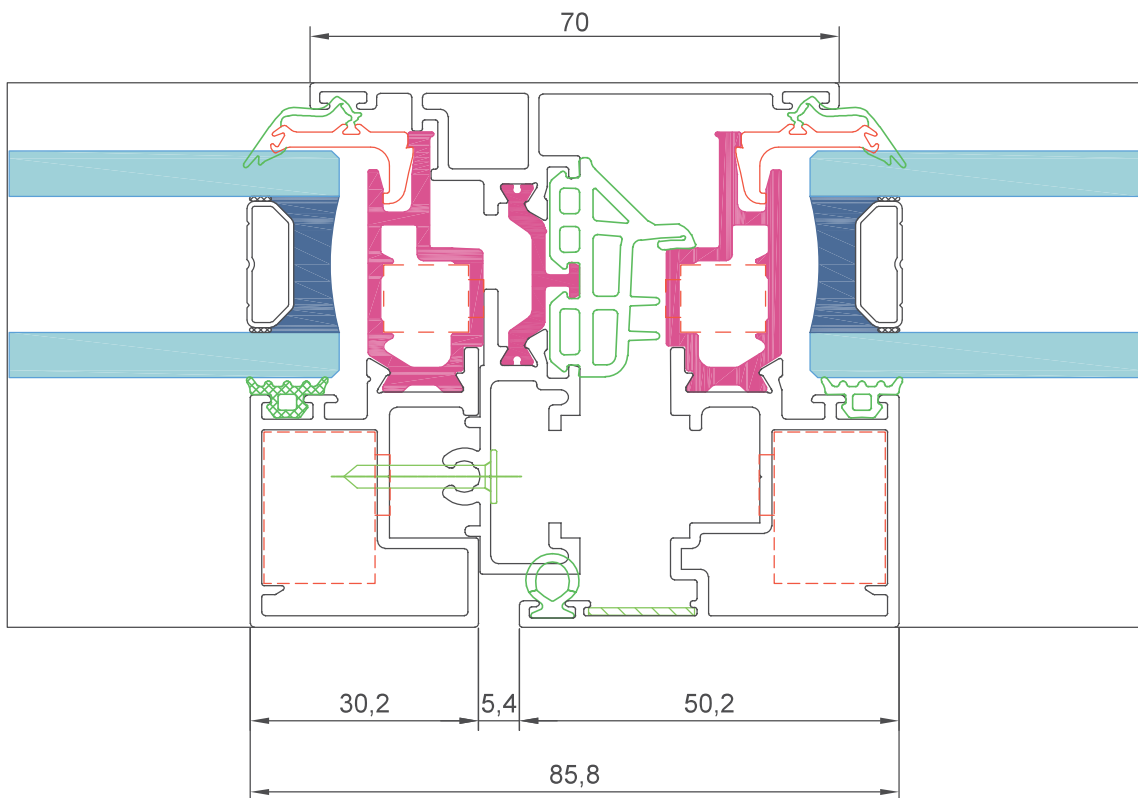
sección 5
