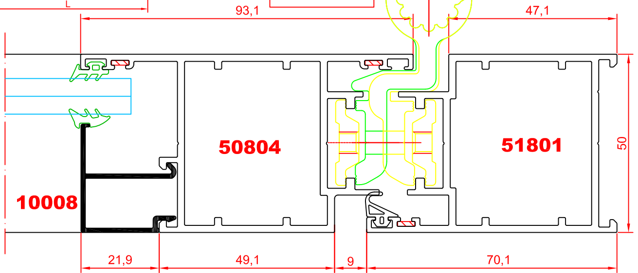
Sección 8
