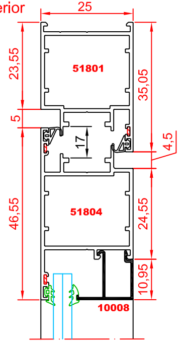
Sección 6 Escala 1:2
