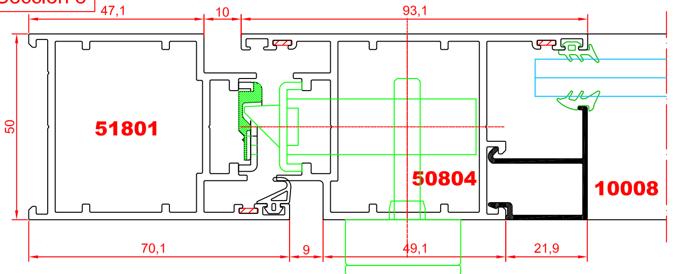
Sección 8
