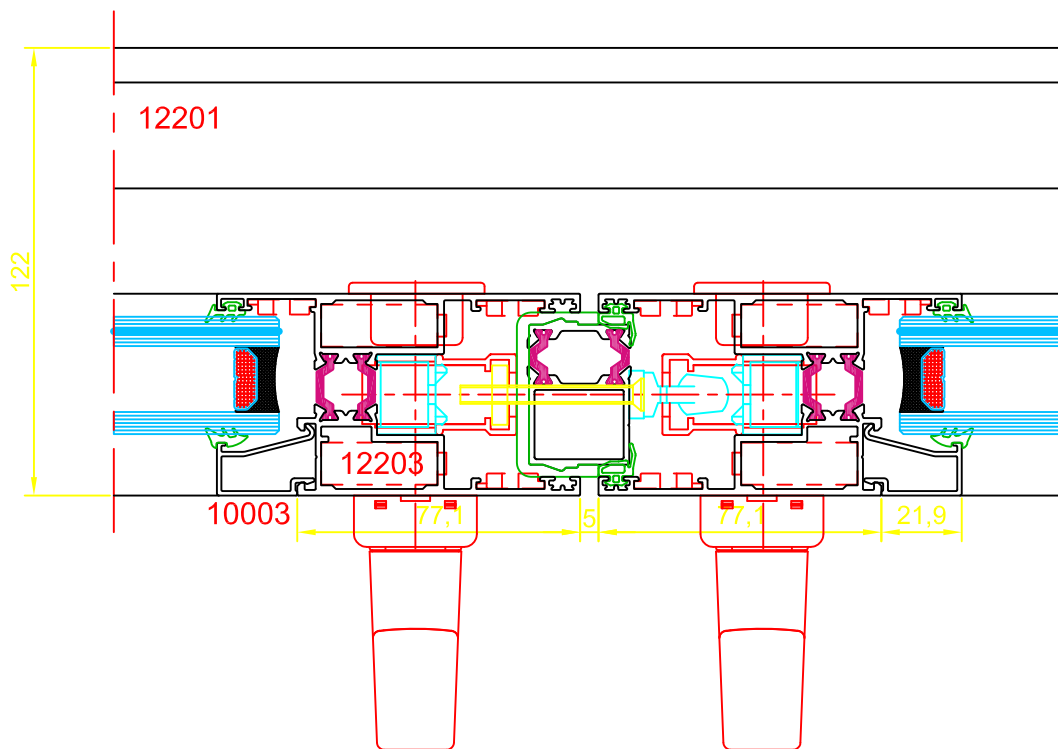
Sección 9 Escala 1:2
